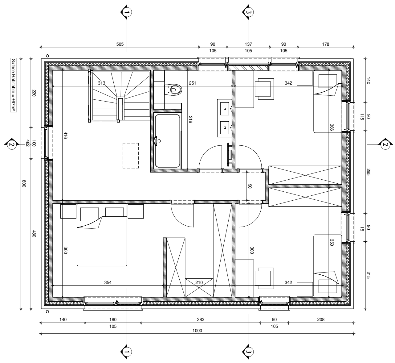
ETAGE
