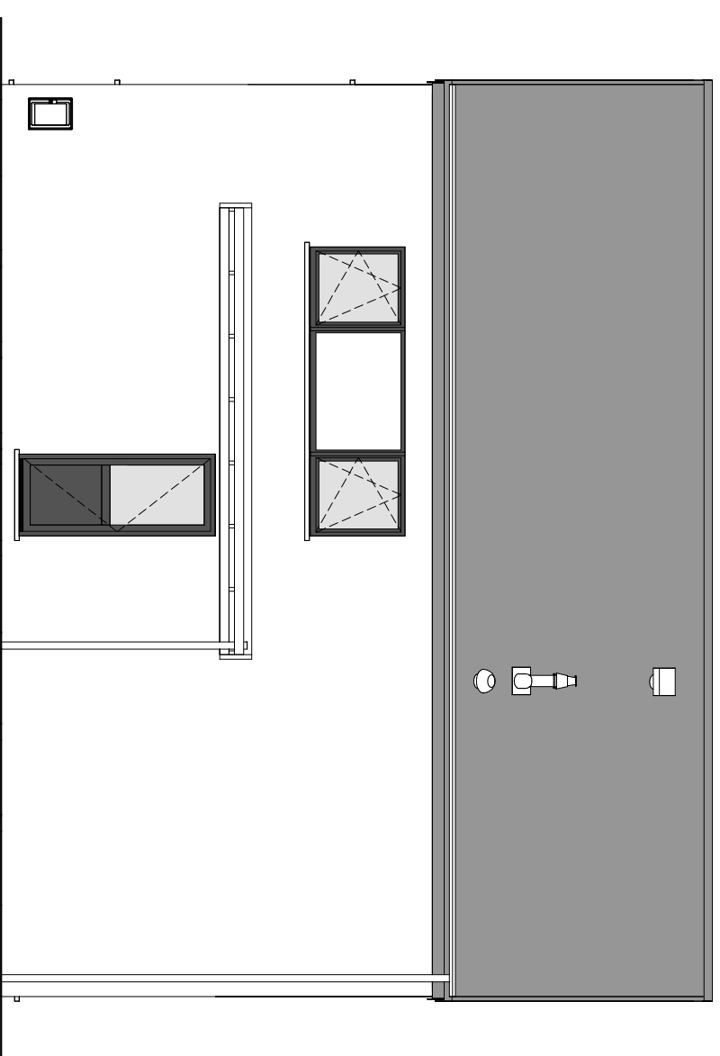
FACADE LATÉRALE GAUCHE
