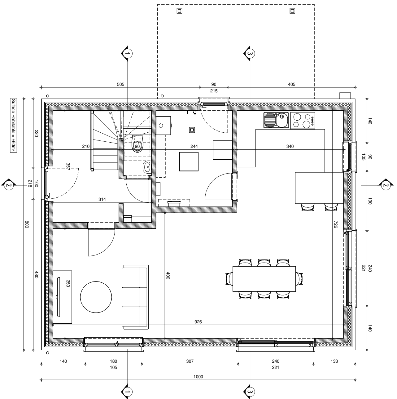
REZ-DE-CHAUSSEE
