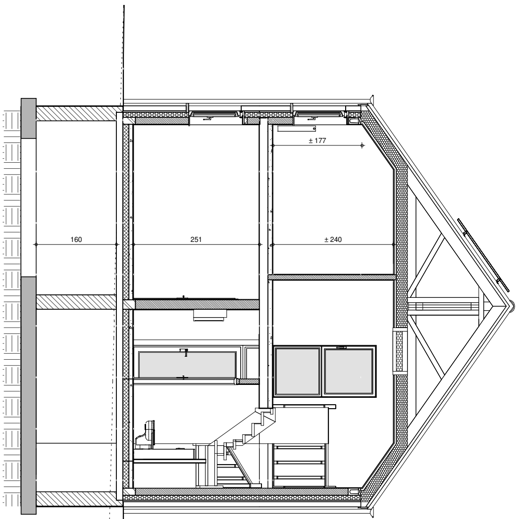
COUPE AA
