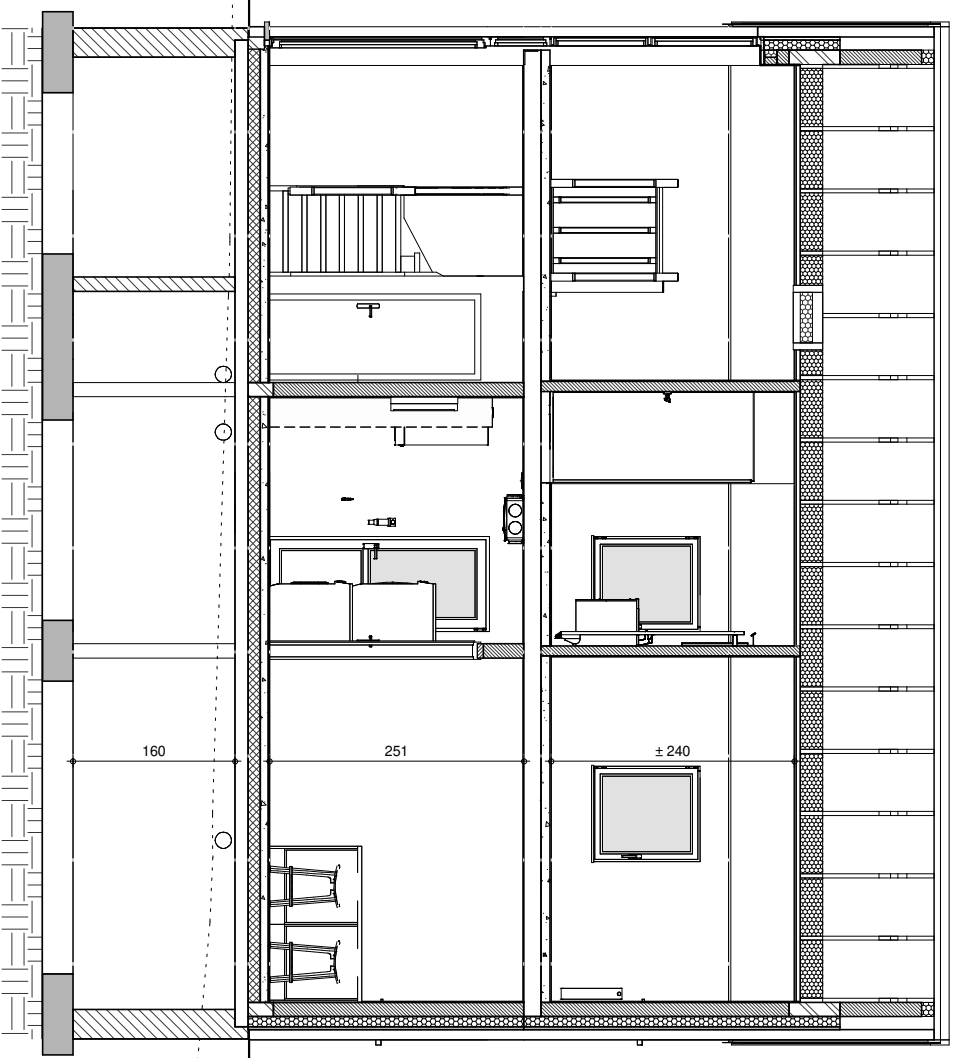
COUPE BB
